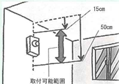
取付可能範囲
