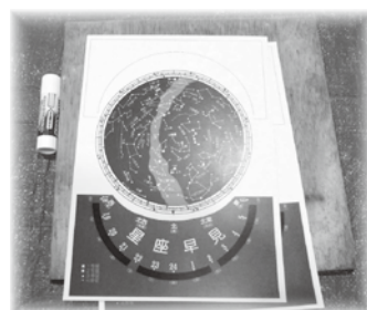
星座早見盤
