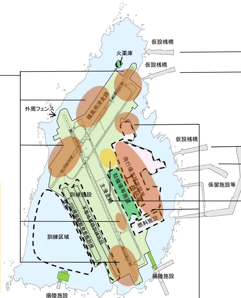
施設全体配置図
